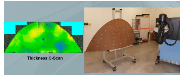
US laser NDT « LUIS » device
